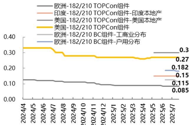
图表10: 各区域组件价格 (USD/W)
